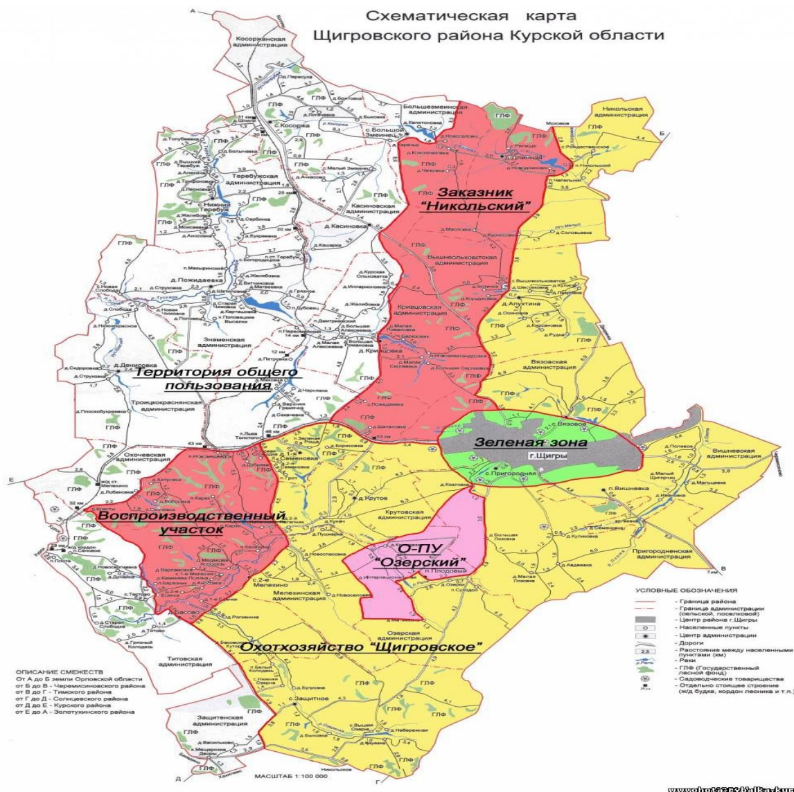
Рисунок 1.4.2.1.3 – Схематическая карта Щигровского района Курской области
